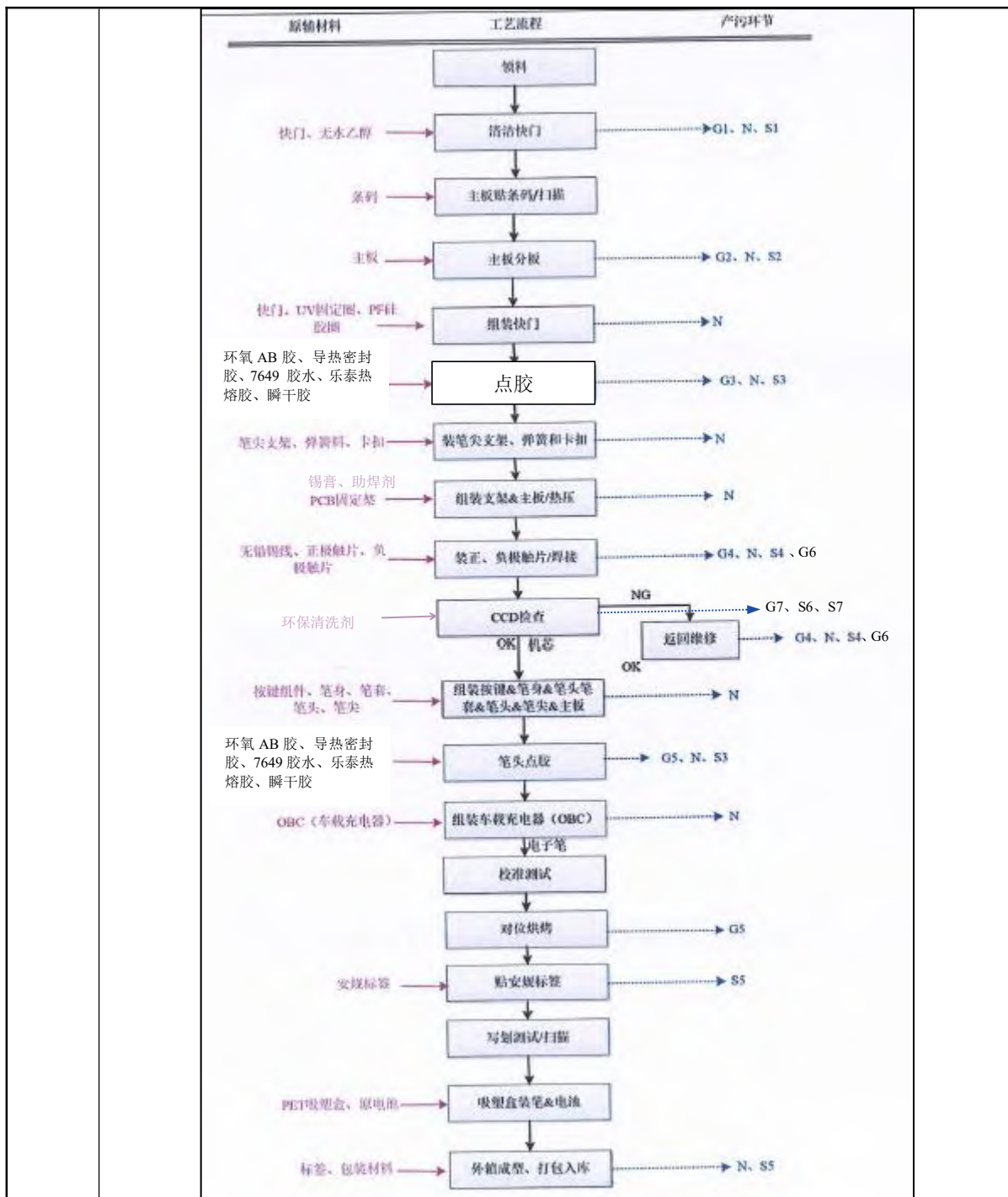
图2-1 项目生产工艺流程及产污环节图
