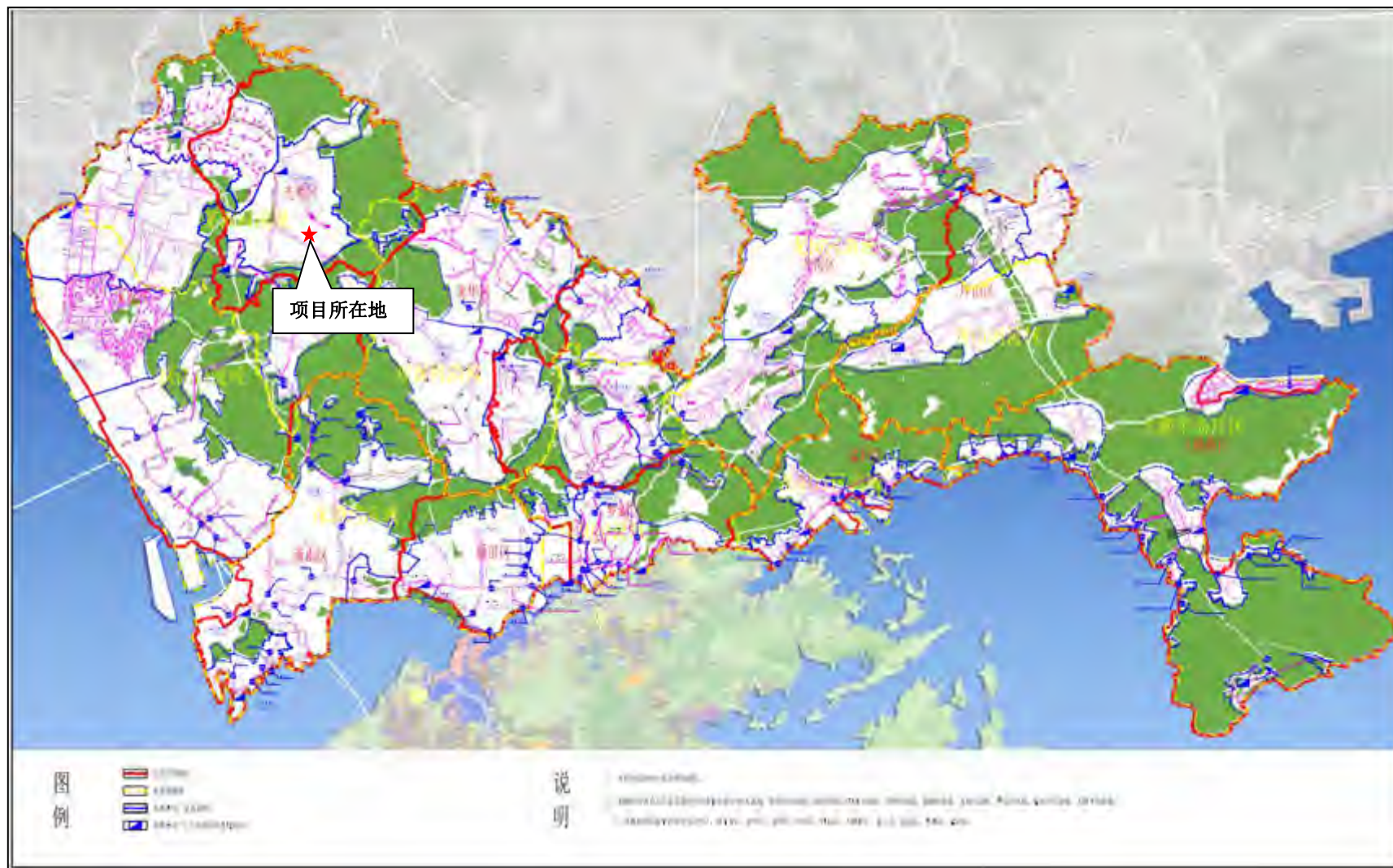
附图 10 项目所在区域污水管网分布图
